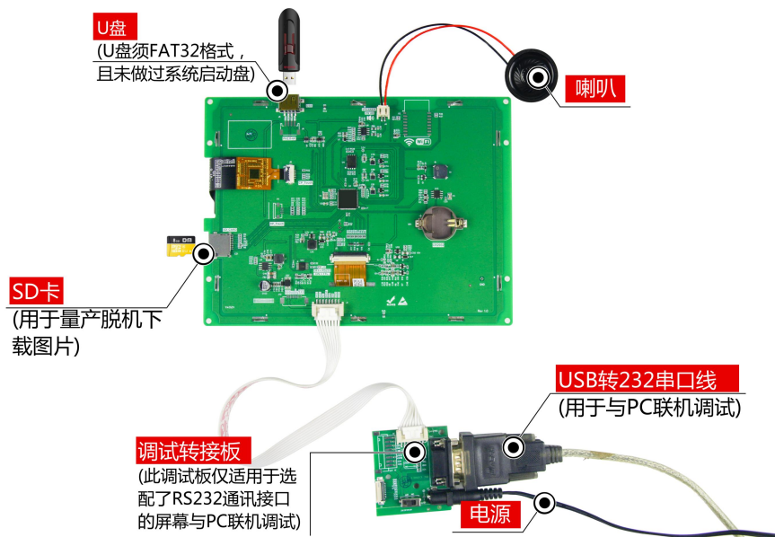
图 1-5 调试工具图
